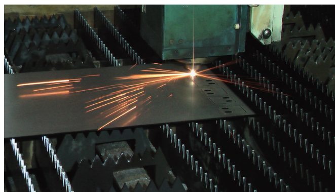
製造工程写真 機械はレーザー切断機
