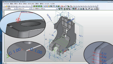
[高精度計測機能]
