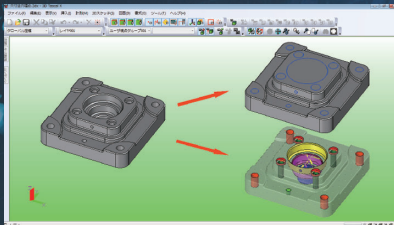
[穴埋め・穴径色分け機能]
