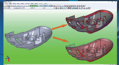
[シャドウ面・肉厚色分け機能]
